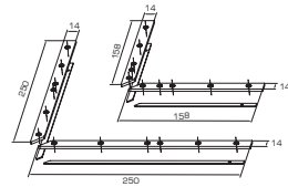
Пластины внешнего углового соединителя
