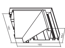
Внутренний угловой соединитель
